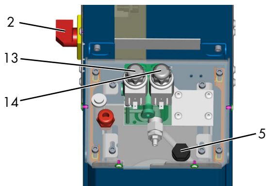
2 interruttore principale 5 apertura di riempimento dell'olio 002 13 valvola V1 14 valvola V2
