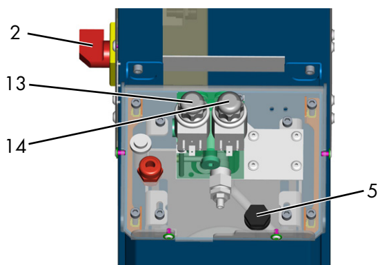
2 Interrupteur principal 13 Vanne V1 002 5 Orifice de remplissage d'huile 14 Vanne V2
