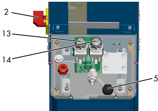
2 Hauptschalter 13 Ventil V1 5 Öleinfüllöffnung 14 Ventil V2 002
